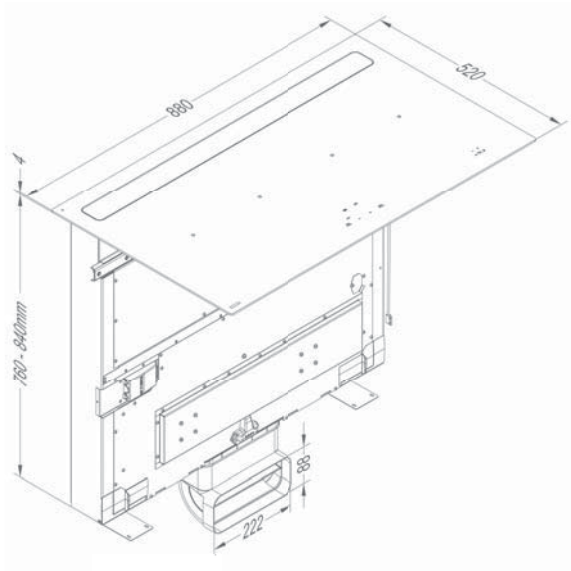
Rysunek 3D
