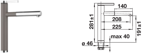
Wylewka obracana o 170°, metalowa osłona węża wylewki
