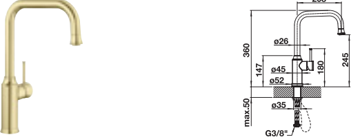
Wylewka obracana o 190°
