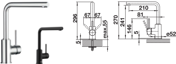
Wylewka obracana o 360° zapewnia większy zasięg
