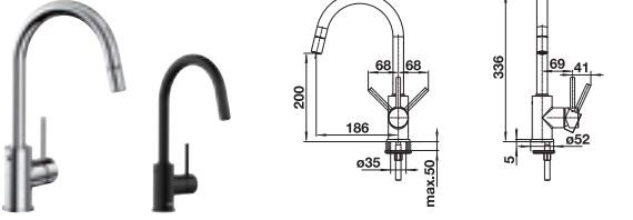
Wylewka obracana o 360° zapewnia większy zasięg
