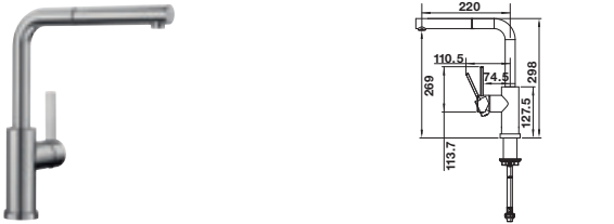
Wylewka obracana o 190°
