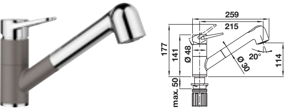
Wylewka obracana o 180°
