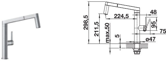
Wylewka obracana o 160°, metalowa osłona węża wylewki
