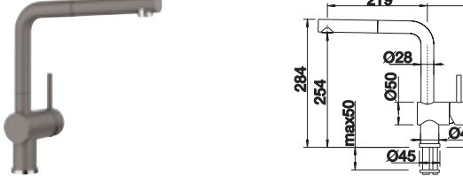
Wylewka obracana o 140°, metalowa osłona węża wylewki
