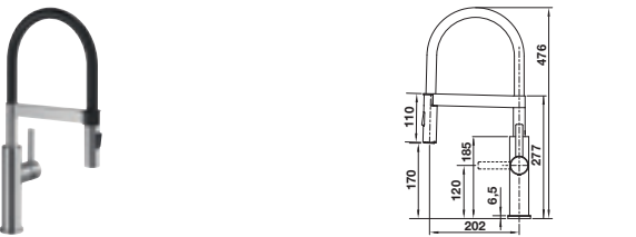
Wylewka obracana o 360° zapewnia większy zasięg, elastyczny czarny wąż zapewnia szeroki zakres ruchu, wylewka z dwoma rodzajami strumienia z łatwym przełączaniem strumienia napowietrzonego na silny strumień prysznicowy, precyzyjny uchwyt magnetyczny zapewnia wygodną blokadę wylewki
