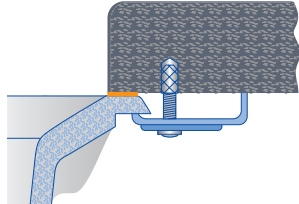
SILGRANIT® PuraDur®: montaż podwieszany zlewozmywaków
