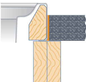
Stal szlachetna: moduł wbudowany między 2 blaty
