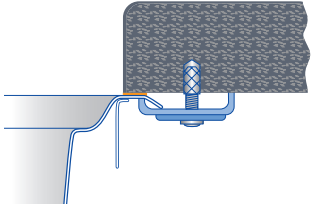
Stal szlachetna: montaż podwieszany zlewozmywaków
