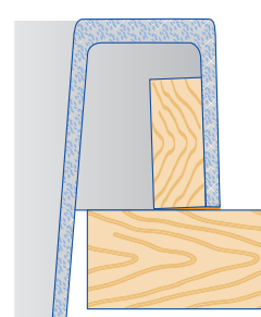
SILGRANIT® PuraDur®: moduł nakładany
