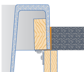
SILGRANIT® PuraDur®: moduł wbudowany między 2 blaty
