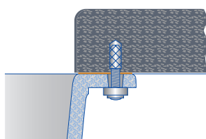
SILGRANIT® PuraDur®: komory podwieszane
