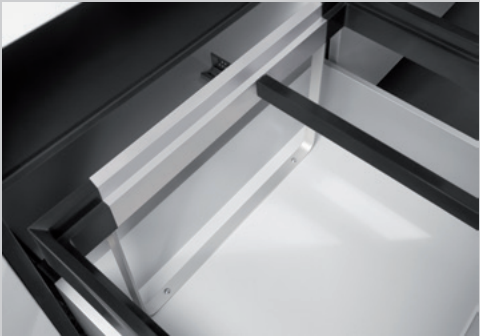
Wysokiej jakości system szufladowy ze wspornikiem mocowanym do dna szuflady wykonany jest z anodowanego aluminium.
